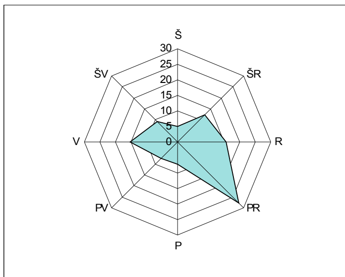
4 pav. Vėjų rožė (vėjo kryptų pasiskirstymas, %) Klaipėdos mieste 2005.11.16 – 2005.12.15
