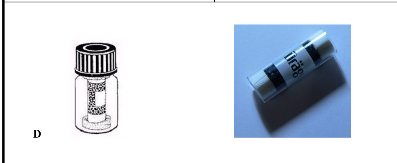
1 pav. Pasyvieji sorbentai ir jų tvirtinimo įrenginys. Apsauginis cilindras skirtas apsaugoti eksponuojamus pasyvius sorbentus nuo kritulių, vėjo, dulkių ir kt. nepalankių veiksnių ( A ). Pasyvieji sorbentai (kaupikliai), skirti oro teršalų koncentracijai aplinkos ore nustatyti: azoto dioksidui ( B ); sieros dioksidui ( C ); lakiesiems organiniams junginiams – benzenui, toluenui, etilbenzenui, ksilenai ( D ).
