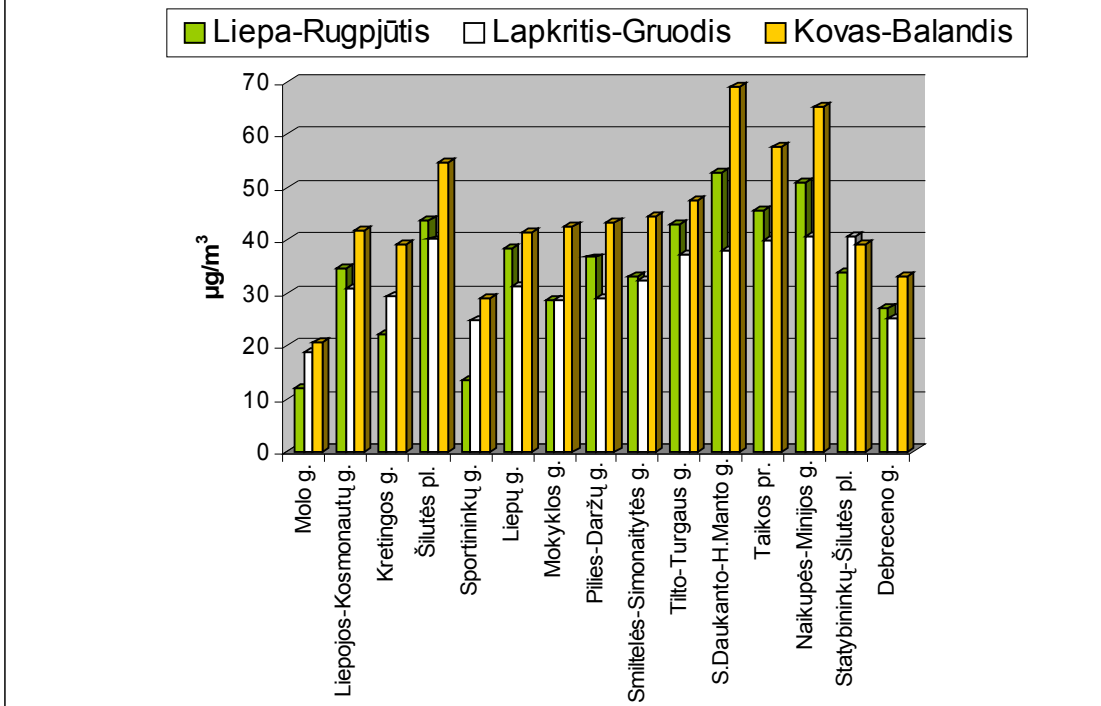
6 pav. Vidutinė NO 2 koncentracija Klaipėdos m. aplinkos ore
