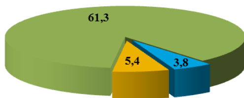
4 pav. 2016 m. stacionarių taršos šaltinių išmestų teršalų kiekis aglomeracijose ir zonoje (tūkstančiai tonų/metus)
