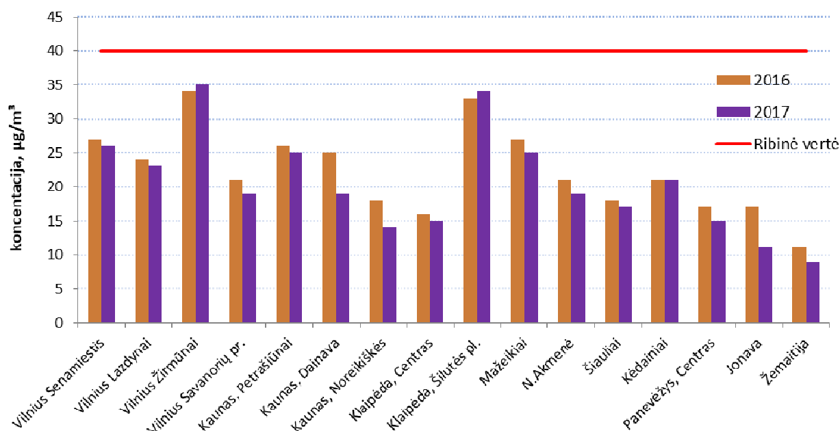
10 pav. Vidutinė metinė KD_{10} koncentracija OKT stotyse 2016–2017 m.
