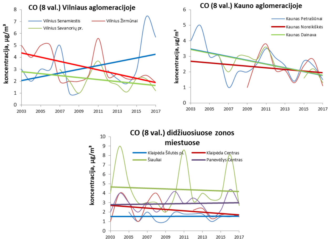
43 pav. Maksimalios 8 val. CO koncentracijos kitimo tendencijos 2003–2017 m.
