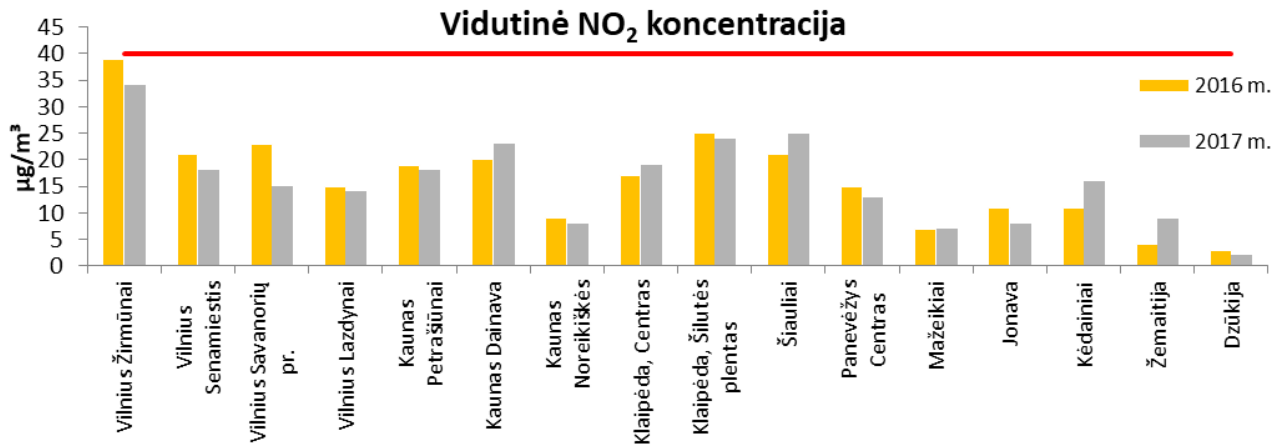
24 pav. Vidutinė metinė NO 2 koncentracija (µg/m 3 ) 2016–2017 m.
