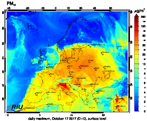
7 pav. Kietųjų dalelių (KD 10 ) pernašos prognozė 2017-10-17 pagal EURAD modelį
