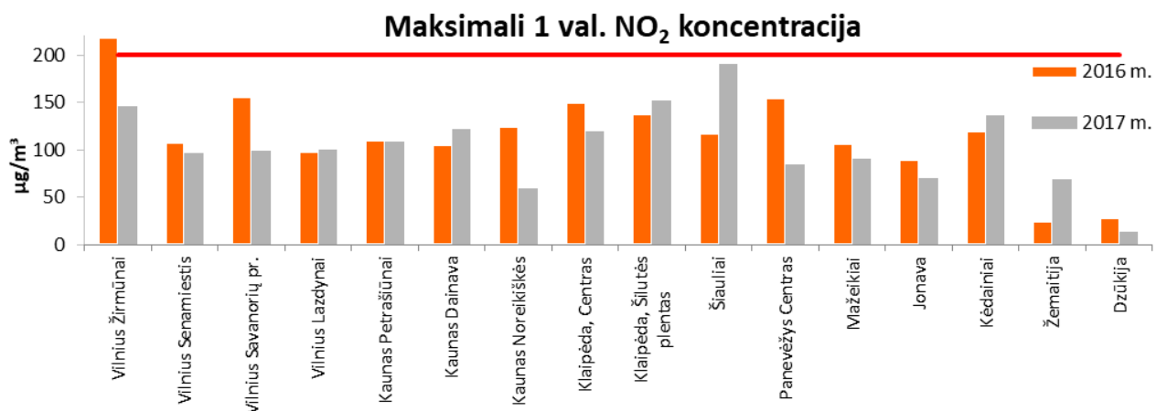
25 pav. Maksimali NO 2 koncentracija (µg/m 3 ) 2016–2017 m.
