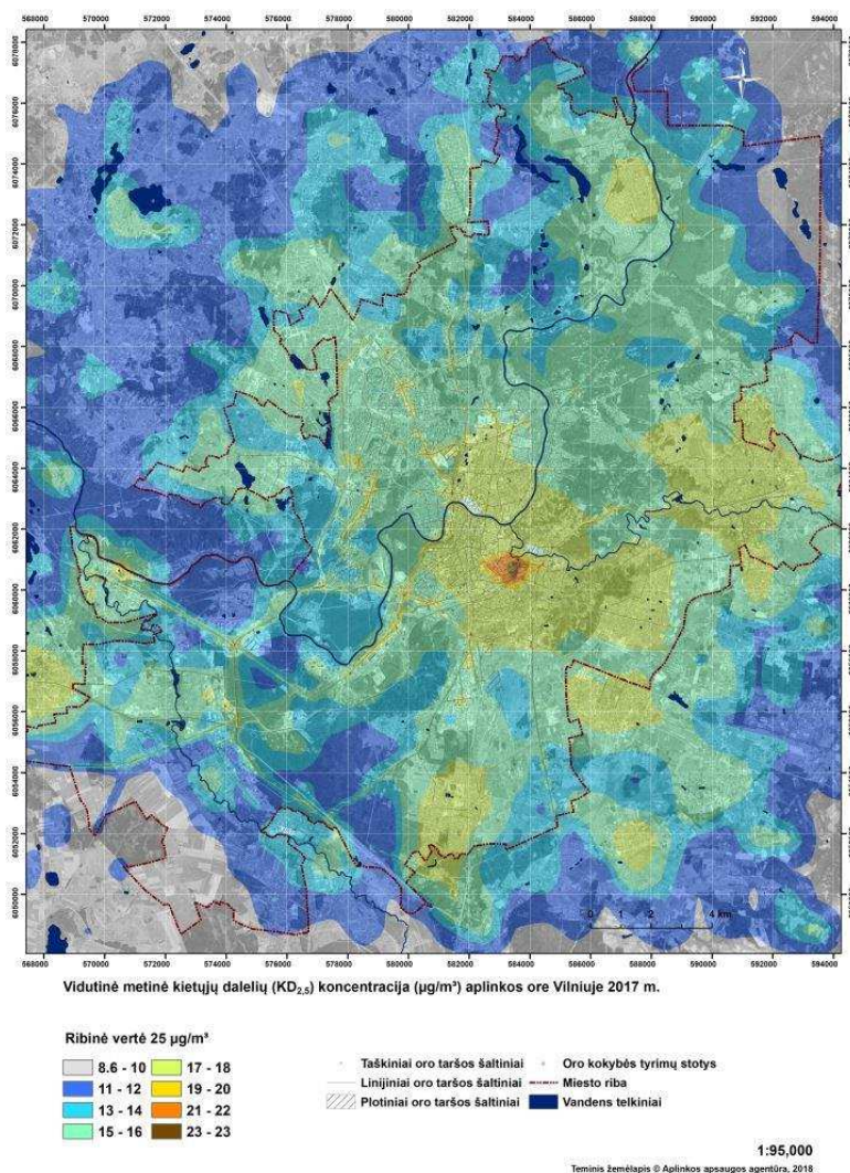
20 pav. Vidutinė metinė \text{KD}_{2,5} koncentracija ( \mu\text{g}/\text{m}^3 ) Vilniuje (pagal ADMS-Urban modelį)
