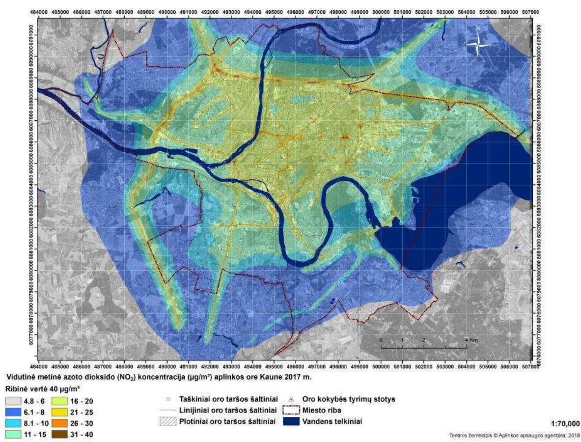
29 pav. Vidutinė metinė NO 2 koncentracija (µg/m 3 ) Kaune (pagal ADMS-Urban modelį)
