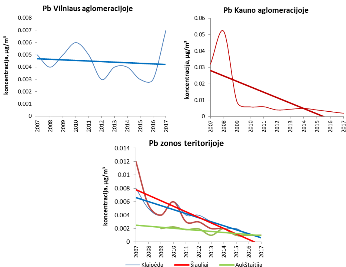
49 pav. Vidutinė Pb koncentracija ir jos kitimo tendencija OKT stotyse 2007-2017 m.
