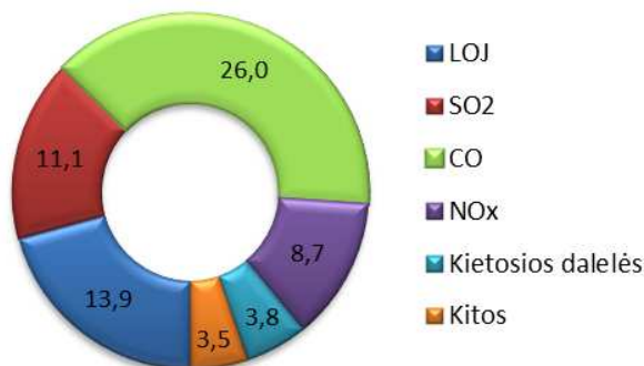
1 pav. Stacionarių taršos šaltinių išmetimai (tūkstančiais tonų) 2017 m.
