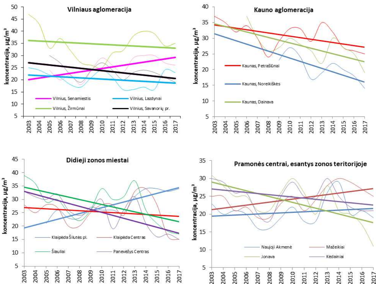
11 pav. Vidutinės metinės KD_{10} koncentracijos kitimo tendencijos 2003–2017 m.
