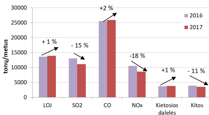
2 pav. 2017 m. išmestų teršalų kiekio pokytis
