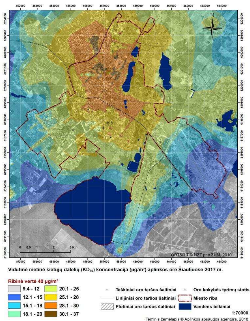
17 pav. Vidutinė metinė KD 10 koncentracija (μg/m 3 ) Šiauliuose (pagal ADMS-Urban modelį)
