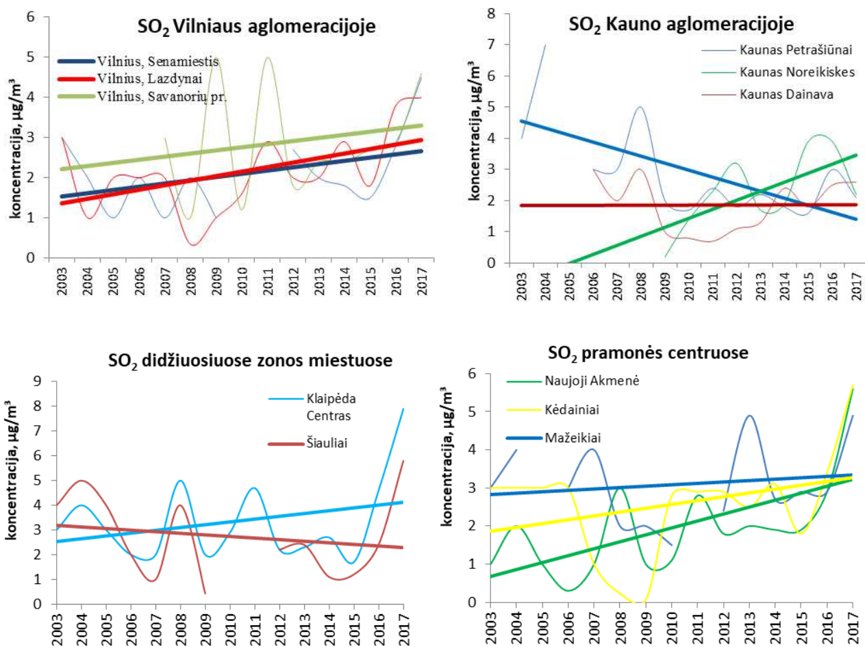
36 pav. Vidutinės metinės SO 2 koncentracijos kitimo tendencijos 2003–2017 m.
