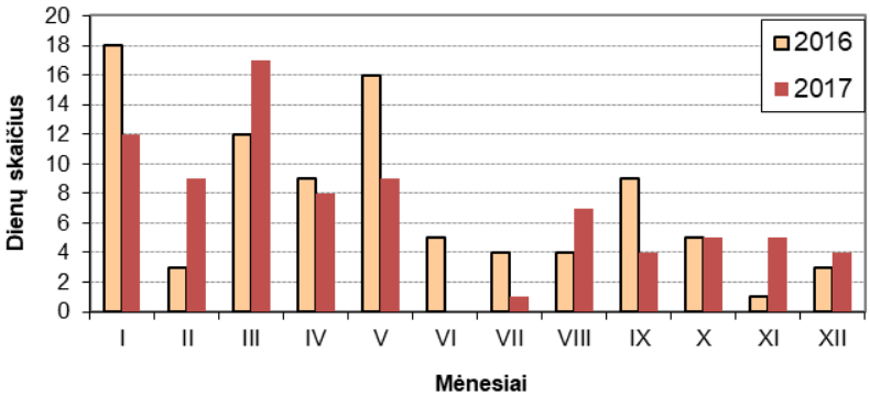
8 pav. Dienų skaičius, kai vyraavo nepalankios teršalų sklaidai meteorologinės sąlygos
