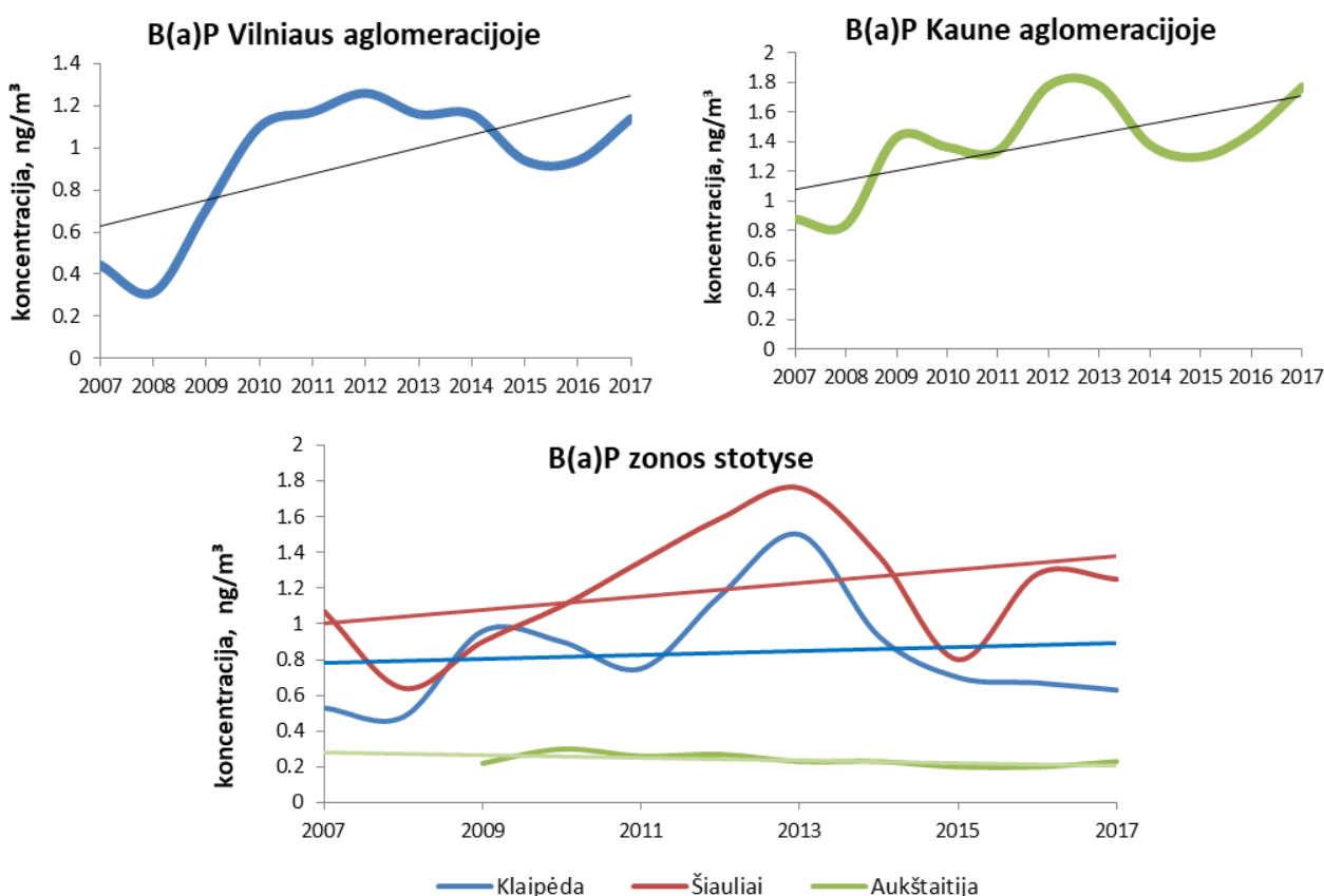
51 pav. Vidutinės metinės B(a)P koncentracijos kitimo tendencijos 2007–2017 m.
