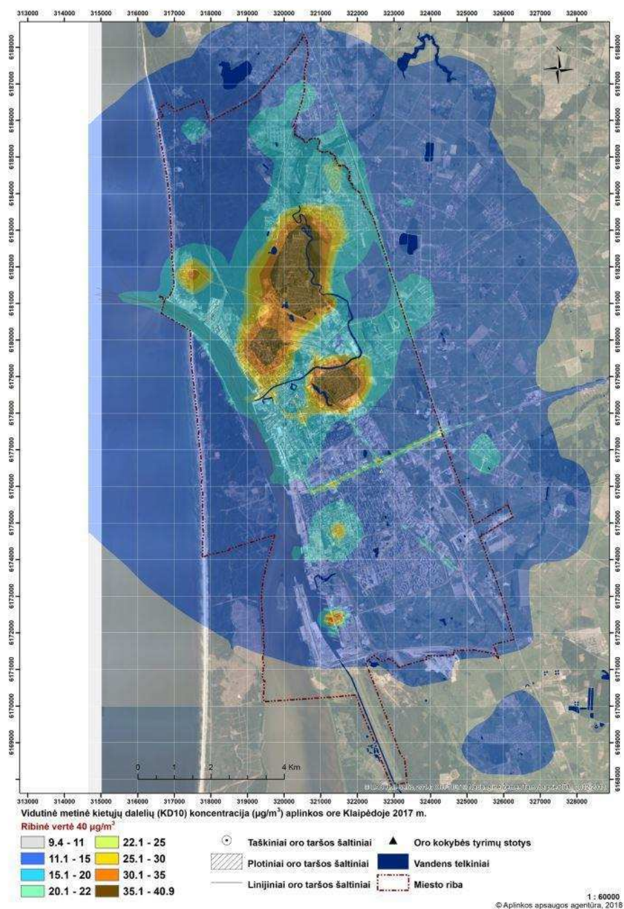
16 pav. Vidutinė metinė KD 10 koncentracija (μg/m 3 ) Klaipėdoje (pagal ADMS-Urban modelį)
