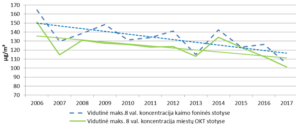
34 pav. Ozono koncentracijos miestų ir kaimo foninėse OKT stotyse kitimo tendencija 2006-2017 m.
