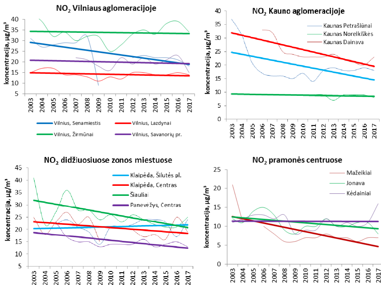
26 pav. Vidutinės metinės NO 2 koncentracijos kitimo tendencijos 2003–2017 m.
