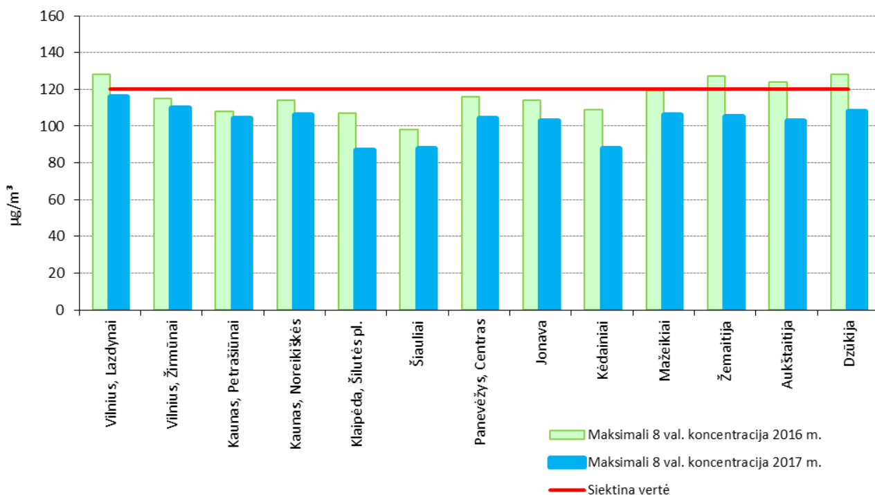
33 pav. Maksimali 8 val. ozono koncentracija 2016-2017 m.
