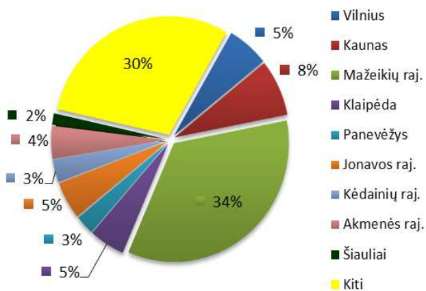
3 pav. 2017 m. stacionarių taršos šaltinių išmestų teršalų kiekis (%)
