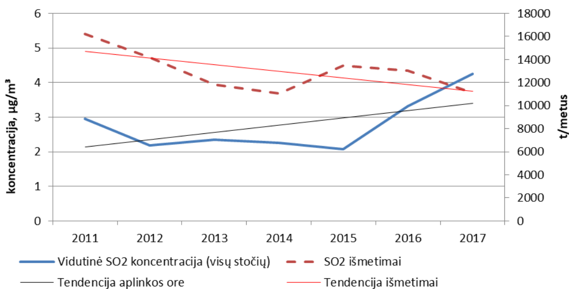
37 pav. Vidutinė metinė SO 2 koncentracija ir sieros dioksido išmetimai iš stacionarių taršos šaltinių
