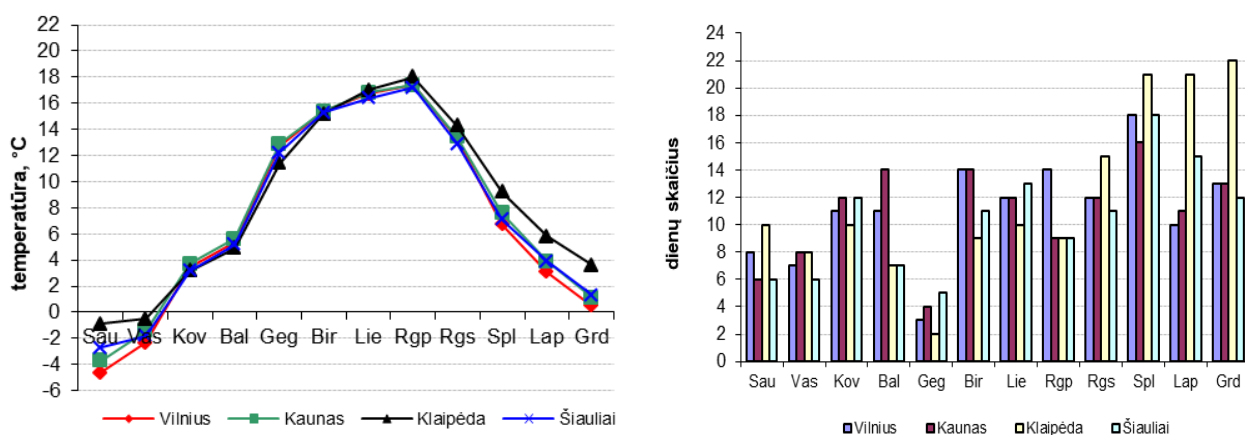
9 pav. Vidutinė mėnesio temperatūra ir dienų su krituliais skaičius Vilniaus, Kauno, Klaipėdos, Šiaulių MS (2017 m.) (Šaltinis: LHMT)
