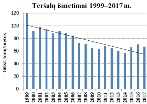
5 pav. Lietuvos teritorijoje išmestų teršalų kiekis (1999–2017 m.) ir jų struktūra (2008–2017 m.)
