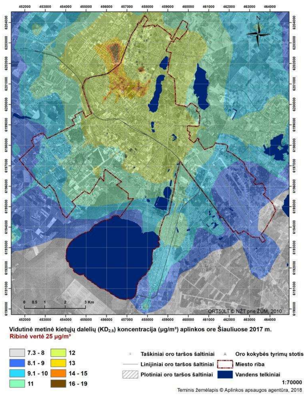
23 pav. Vidutinė metinė KD 2,5 koncentracija (µg/m 3 ) Šiauliuose (pagal ADMS-Urban modelį)
