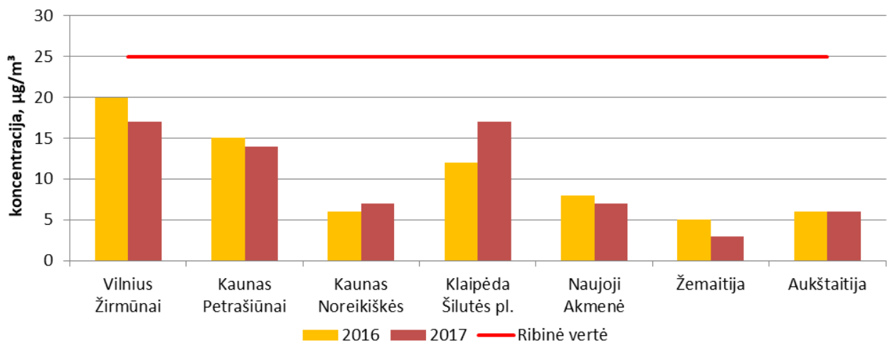
18 pav. Vidutinė metinė kietųjų dalelių KD_{2,5} koncentracija OKT stotyse 2016-2017 m.
