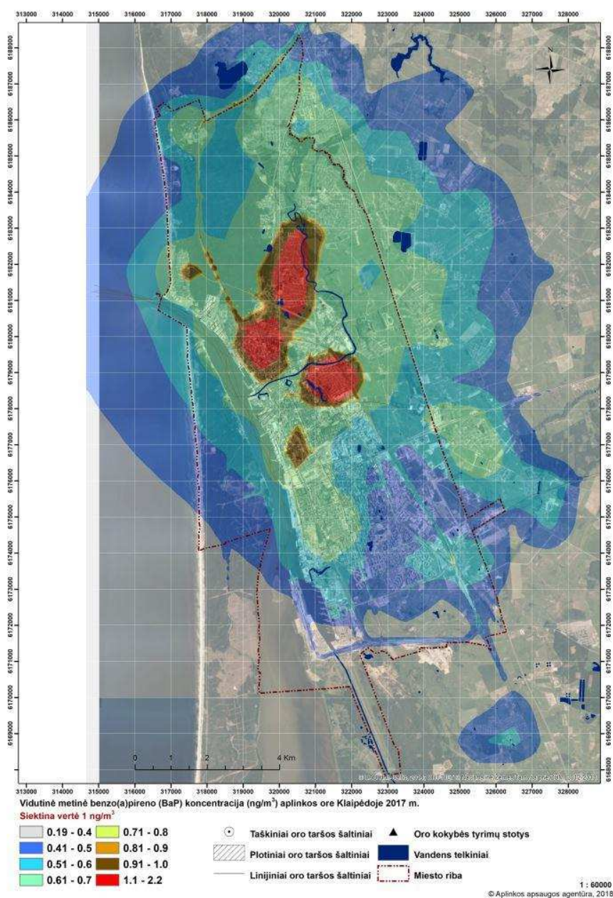
54 pav. Vidutinė metinė B(a)P koncentracija (ng/m 3 ) Klaipėdoje (pagal ADMS Urban modelį)
