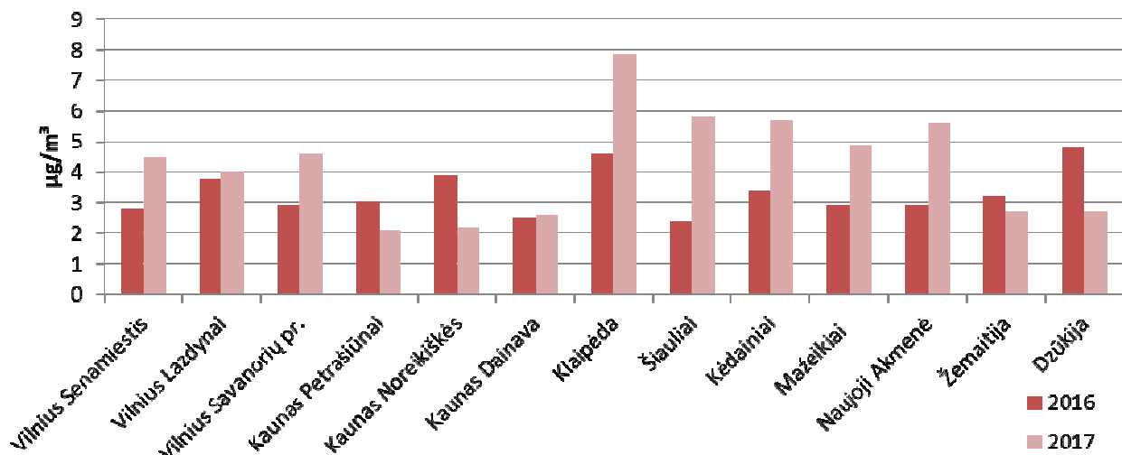
35 pav. Vidutinė metinė SO 2 koncentracija (µg/m 3 ) 2016–2017 m.
