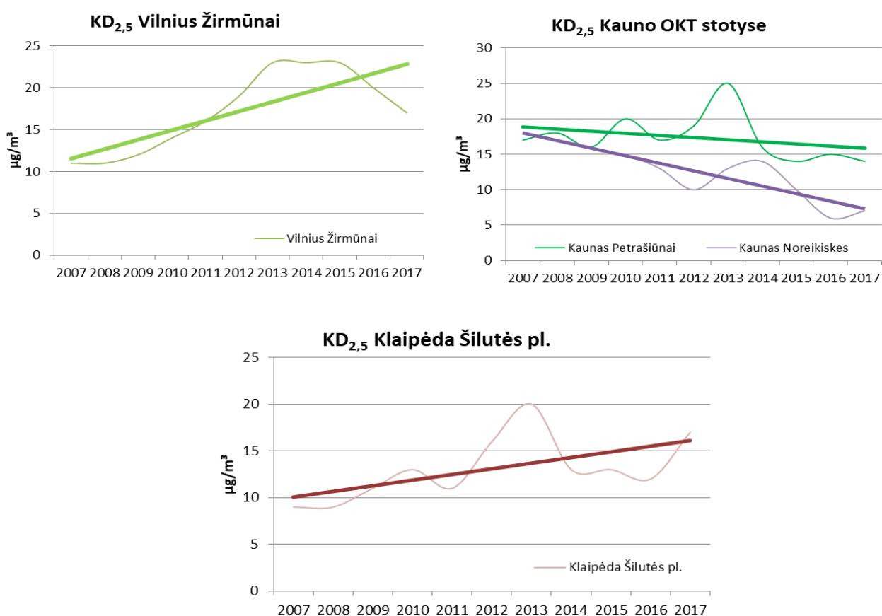
19 pav. Vidutinės metinės KD_{2,5} koncentracijos kitimo tendencijos 2007–2017 m.
