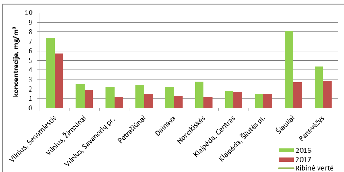
42 pav. Maksimali 8 val. anglies monoksido koncentracija OKT stotyse 2016-2017 m.
