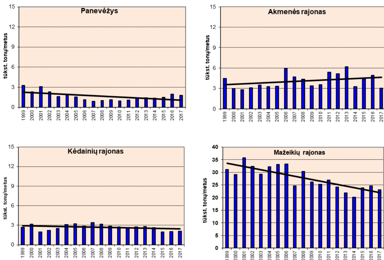
6 pav. Stacionarių taršos šaltinių į atmosferą 1999-2017 m. išmestų teršalų kiekis (tūkst. t/m) ir jo kitimo tendencija didžiausiuose šalies miestuose ir pramonės rajonuose
