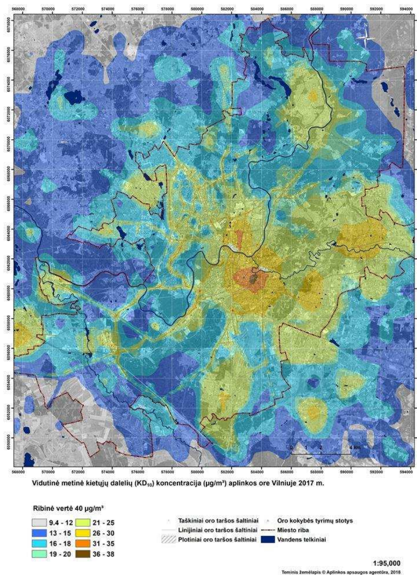
14 pav. Vidutinė metinė KD 10 koncentracija (µg/m 3 ) Vilniuje (pagal ADMS-Urban modelį)
