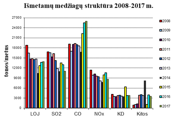
5 pav. Lietuvos teritorijoje išmestų teršalų kiekis (1999–2017 m.) ir jų struktūra (2008–2017 m.)
