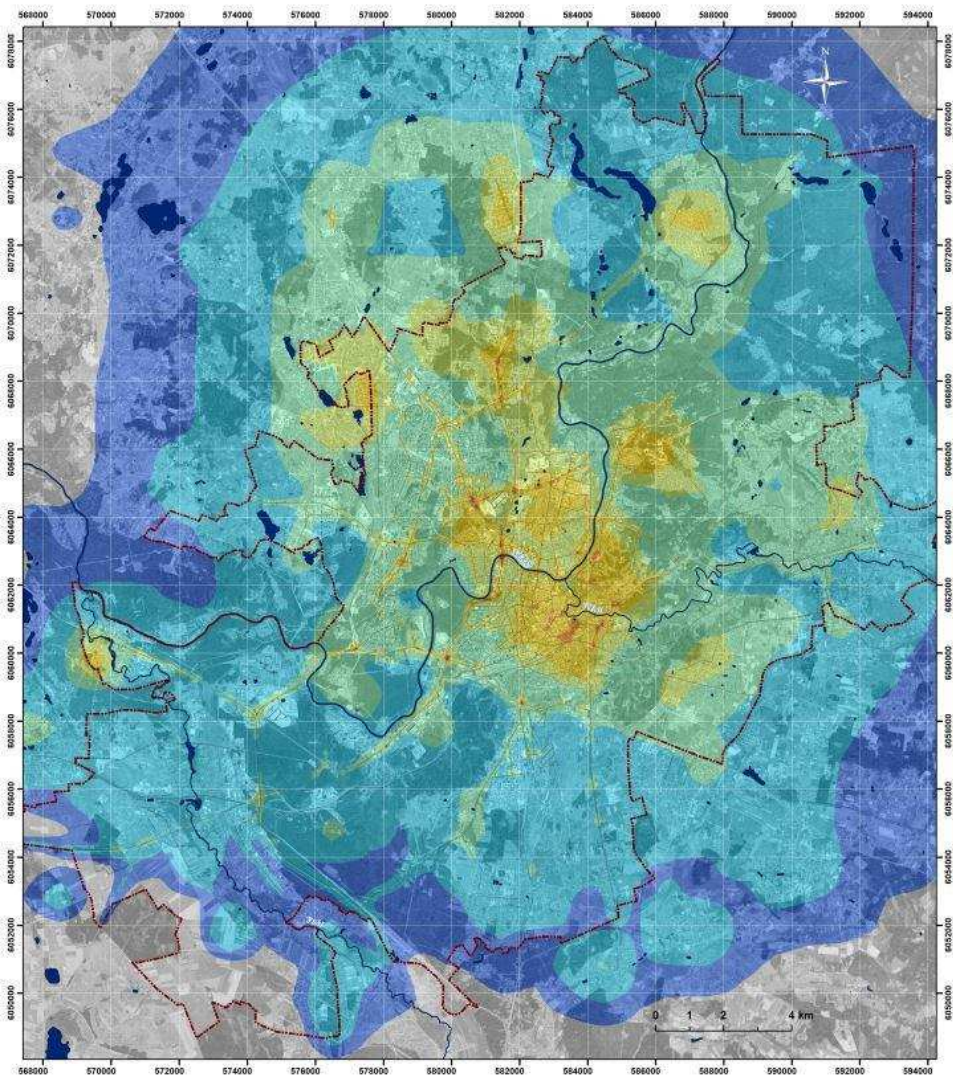
Vidutinė metinė anglies monoksido (CO) koncentracija (mg/m 3 ) aplinkos ore Vilniuje 2017 m.
