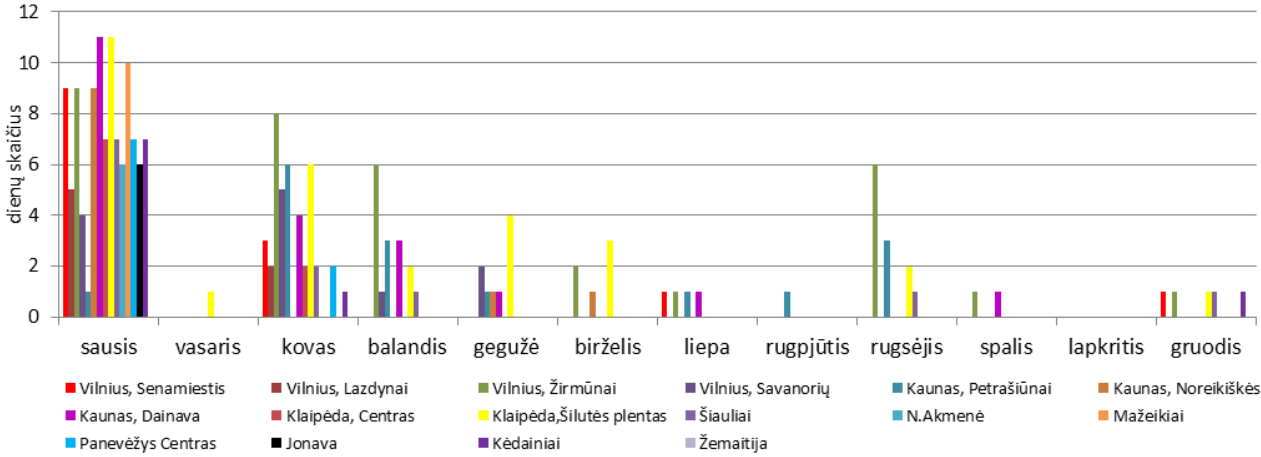
12 pav. Dienų skaičius atskirais mėnesiais, kai buvo viršyta KD 10 koncentracijos paros ribinė vertė 2017 m.
