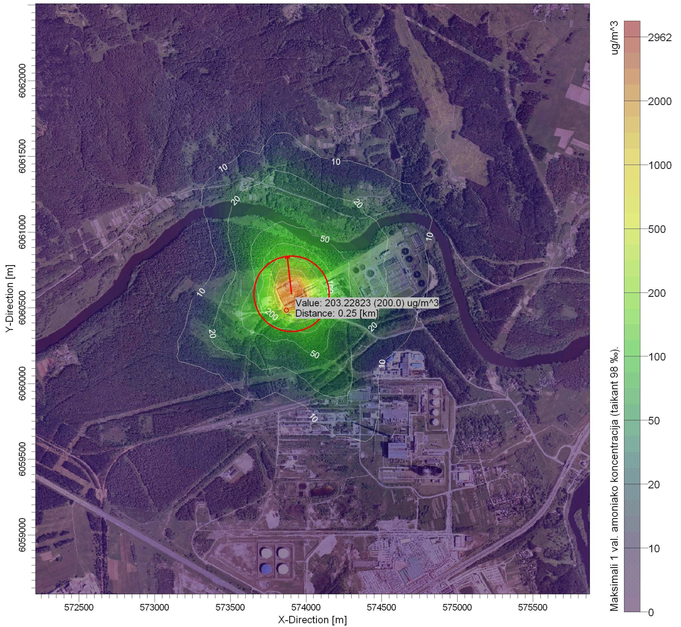
1 pav. Amoniako sklaidos vaizdas, kai emisija yra 44,8 t/metus arba 0,000058 g/s/ \text{m}^2 , esant 2,5 ha paviršiniam šaltiniui.
